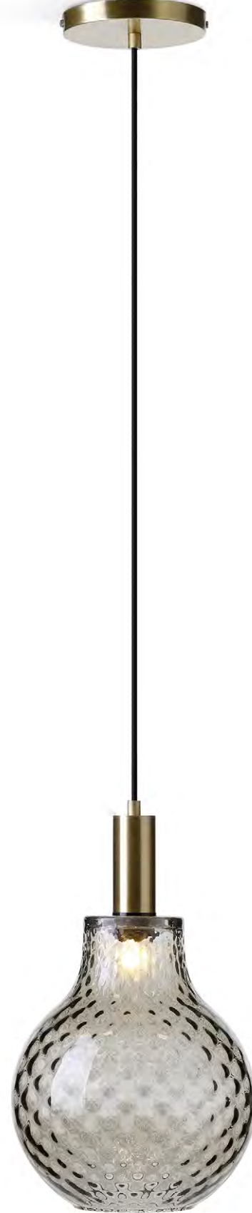
AR3238 Dimensões/Dimensions 100cm - 15cm Dimensões tubo/Tube dimension 40mm Materiais/Materials Latão escovado e vidro/Brushed brass and glass
